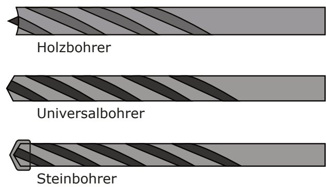
Bohrer
