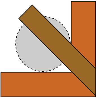
Zentrumsanreisser um das Zentrum von einem Rad anzuzeichnen
